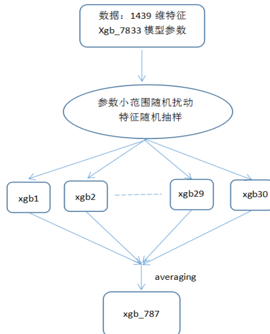
图 11. Xgb 模型 bagging
